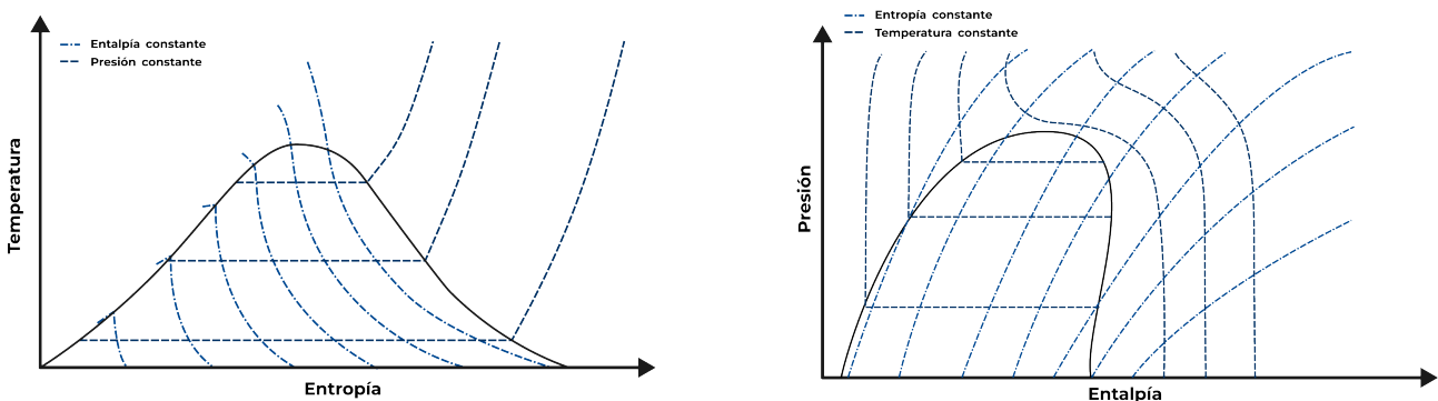
Figura 1.11: Diagramas de T-s y p-h y sus curvas de propiedades constantes.
