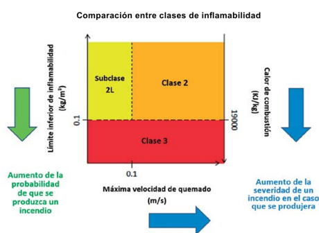
Figura 1.10: Comparación entre clases de inflamabilidad.
