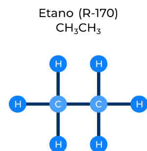
Figura 1.5: Molécula de etano.
